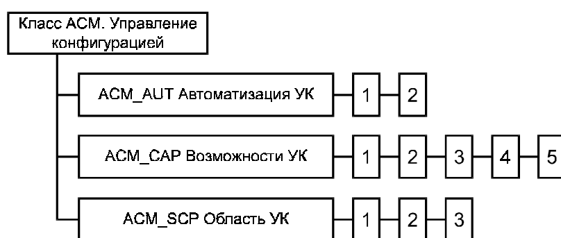
Рисунок 8.1 — Декомпозиция класса «Управление конфигурацией»
